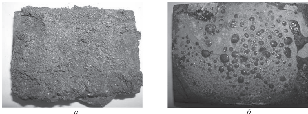
Рис. 4. Исследование наплавляемости: а – исходная дробь ДЧЛ 08; б – диффузионно-легированная дробь ДЧЛ 08
