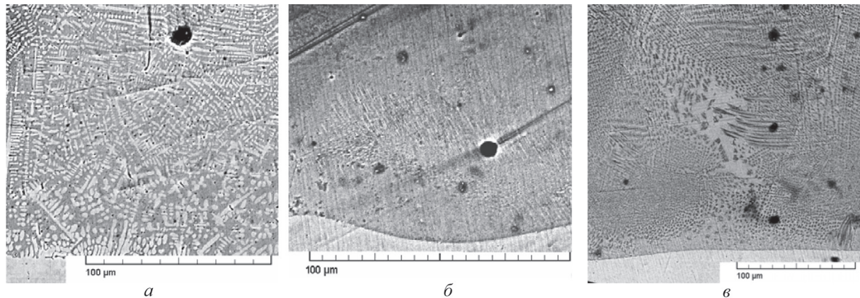
Рис. 3. Структура МЭУ-покрытий: из чугуна борированной дроби (а – доэвтектическая; б – эвтектическая; в – заэвтектическая)
