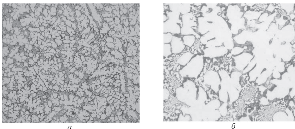
Рис. 5. Микроструктура слоя после наплавки смеси с борированной ДЧЛ 08: а – \times 200 ; б – \times 1000
