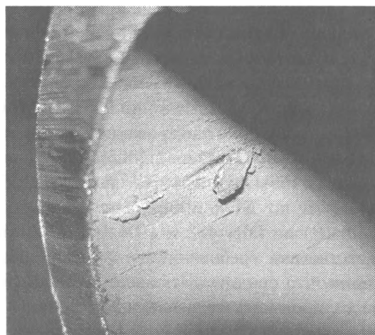
Рис. 1. Сталеплавильная пленка на внутренней поверхности трубы
