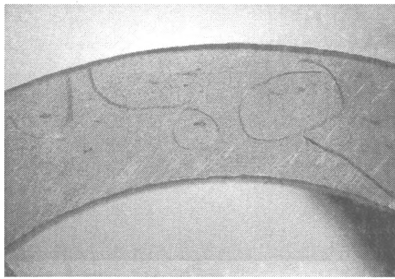
Рис. 5. Макровключения в поперечном сечении трубы
