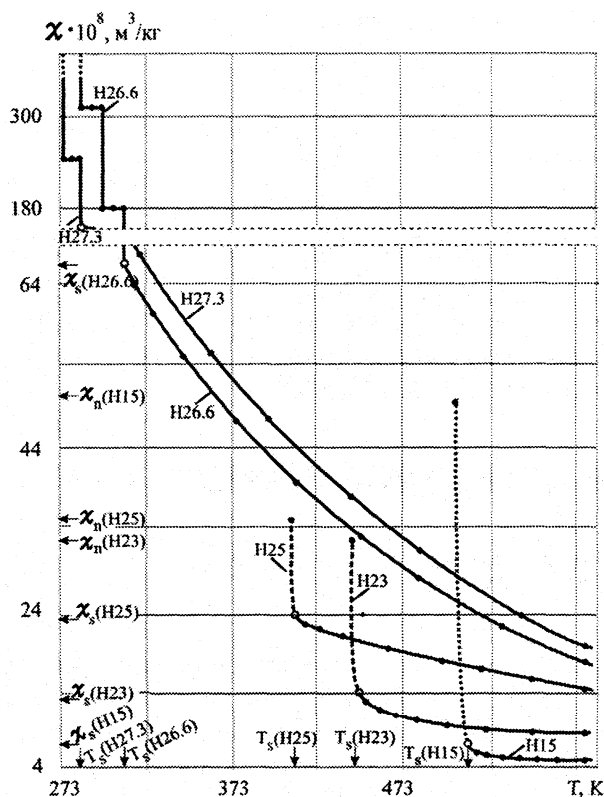
Рис. 1. Типичные температурные зависимости удельной магнитной восприимчивости \chi ( H = 0,2 \cdot 10^6 А/м) Fe – Ni-сплавов с выдержкой в точках T_s . Стрелками показаны стартовые (с индексом s) и конечные (с индексом n) значения \chi в точке T_s
