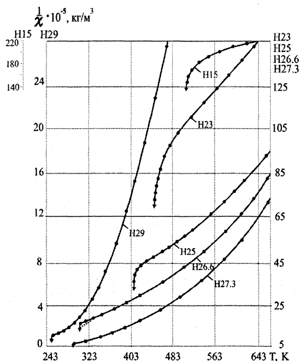
Рис. 3. Типичные температурные зависимости обратной удельной восприимчивости Fe – Ni-сплавов
