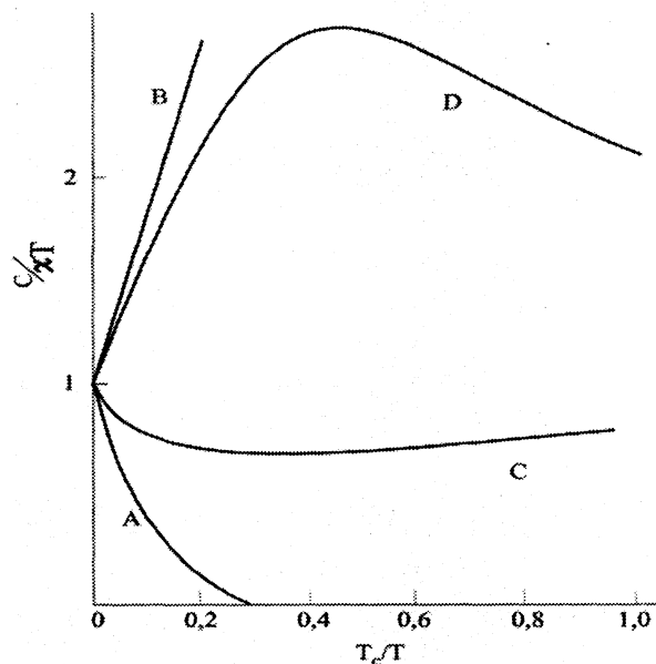
Рис. 2. Зависимости C/\chi T от приведенной температуры, полученные в [5]
