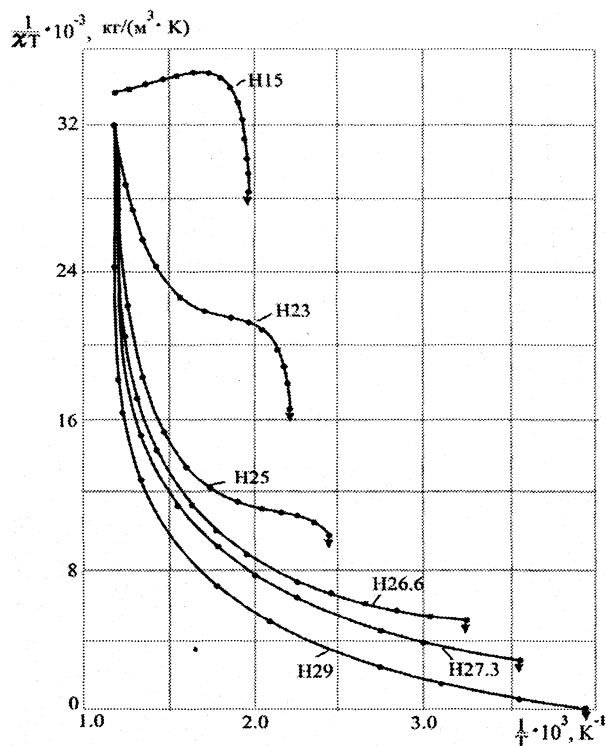
Рис. 4. Зависимость \frac{1}{\chi T} \left( \frac{1}{T} \right) для Fe – Ni-сплавов
