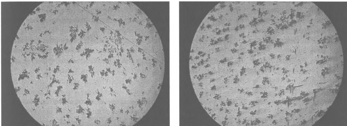
Рис. 3. Микроструктура ковкого чугуна после отжига в течение 12 ч: a – с добавкой 0,015% Al; б – с добавкой 0,015% Al + 0,042% Bi-Mo отработанного катализатора. \times 500
