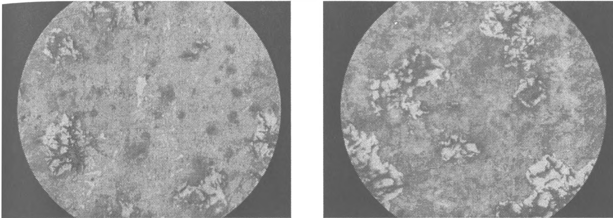
Рис. 3. Микроструктура ковкого чугуна после отжига в течение 12 ч: a – с добавкой 0,015% Al; б – с добавкой 0,015% Al + 0,042% Bi-Mo отработанного катализатора. \times 500
