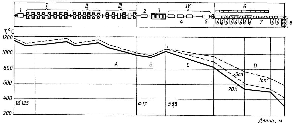
Рис. 2. Расчет изменения средней температуры раската на стане 320/150: I — гидросбив окалины; 2 — водяное охлаждение; 3 — Морган-блок; 4, 5 — секции водяного охлаждения; 6 — изолирующие крышки; 7 — трасса воздушного охлаждения (Стелмор); 8 — бунтоприемник: I — черновая группа клетей; II — промежуточная группа клетей; III — чистовые клетки; IV — трасса водовоздушного охлаждения
