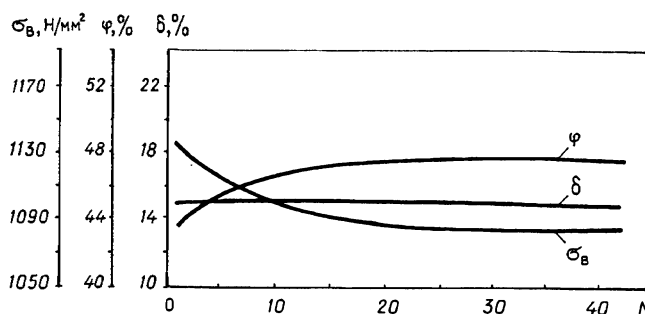
Рис. 5. Распределение механических свойств катанки по длине лотка. N — номер витка от начала мотка
