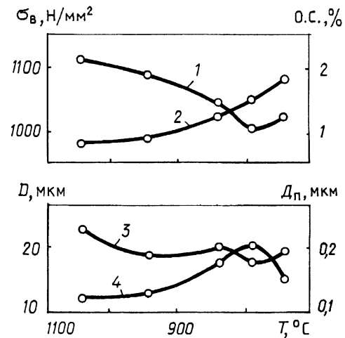
Рис. 3. Зависимость \sigma_b (1), (О.С.) (2), D (3), D_p (4) в катанке из стали 70К от среднemasсовой температуры после ускоренного охлаждения
